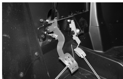
Педаль газа
