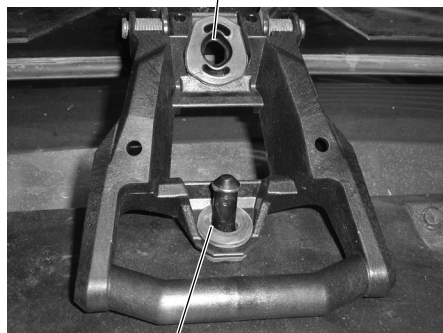
Заднее кольцо (фиксирует открытое стекло)
