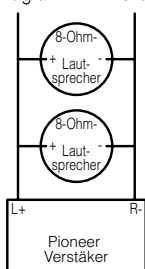
4-Ohm-Überbrückungsmodus
