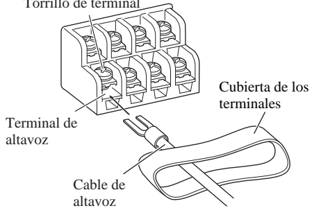
Torrillo de terminal
