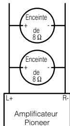
Branchement en pont de 8 Ω
