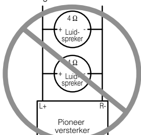
2 \Omega brugschakeling
