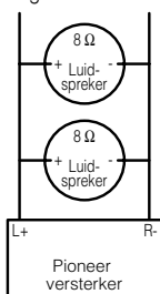
4 \Omega brugschakeling
