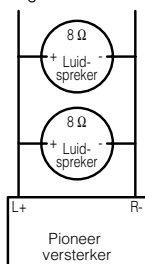
4 Ω brugschakeling
