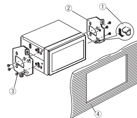
① Подогните зажим, если он мешает установке. ② Заводской установочный кронштейн ③ Используйте винты либо с круглыми (5 мм × 8 мм), либо с плоскими головками (5 мм × 9 мм), в зависимости от формы отверстий под винты кронштейна. ④ Приборная панель или консоль
