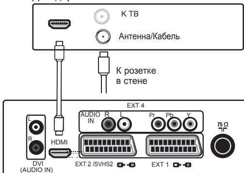
Разъемы внизу телевизора
