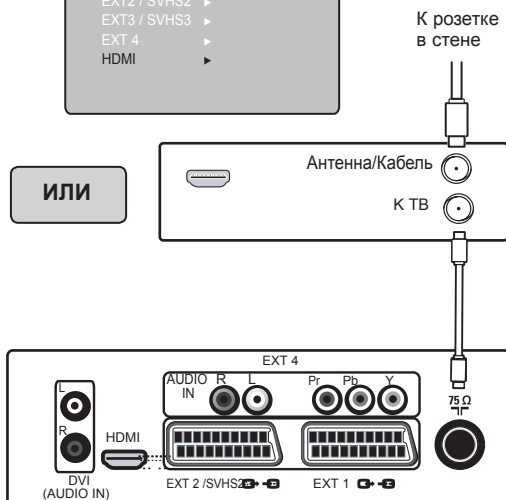
Разъемы внизу телевизора
