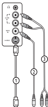
Разъемы сбоку телевизора
