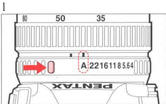
1. УСТАНОВКА ЗНАЧЕНИЯ ДИАФРАГМЫ НА ОБЪЕКТИВЕ
