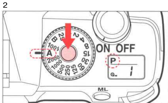
2. УСТАНОВКА ЗНАЧЕНИЯ ВЫДЕРЖКИ НА ФОТОКАМЕРЕ
