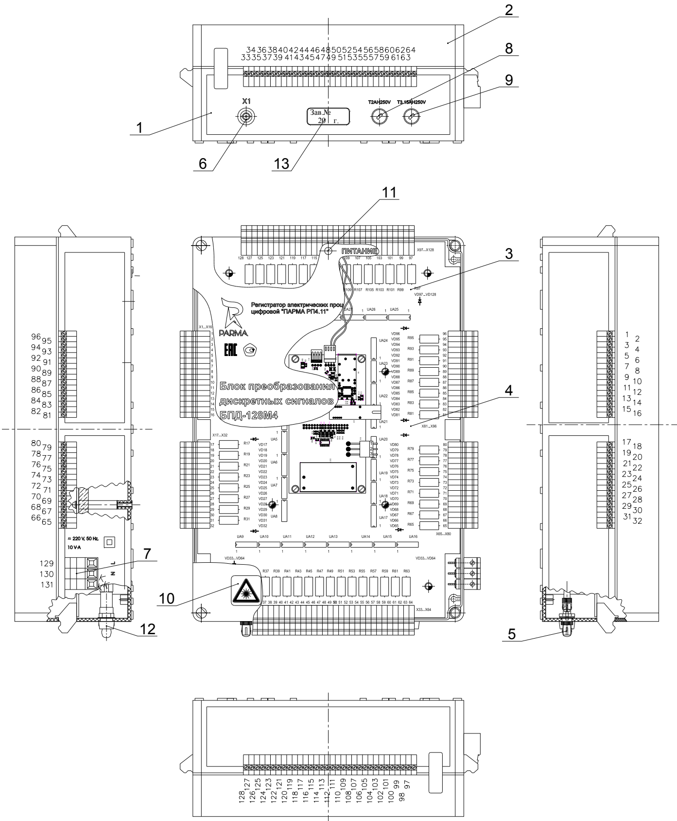
Рисунок 3- Внешний вид и устройство блока БПД-128М4
