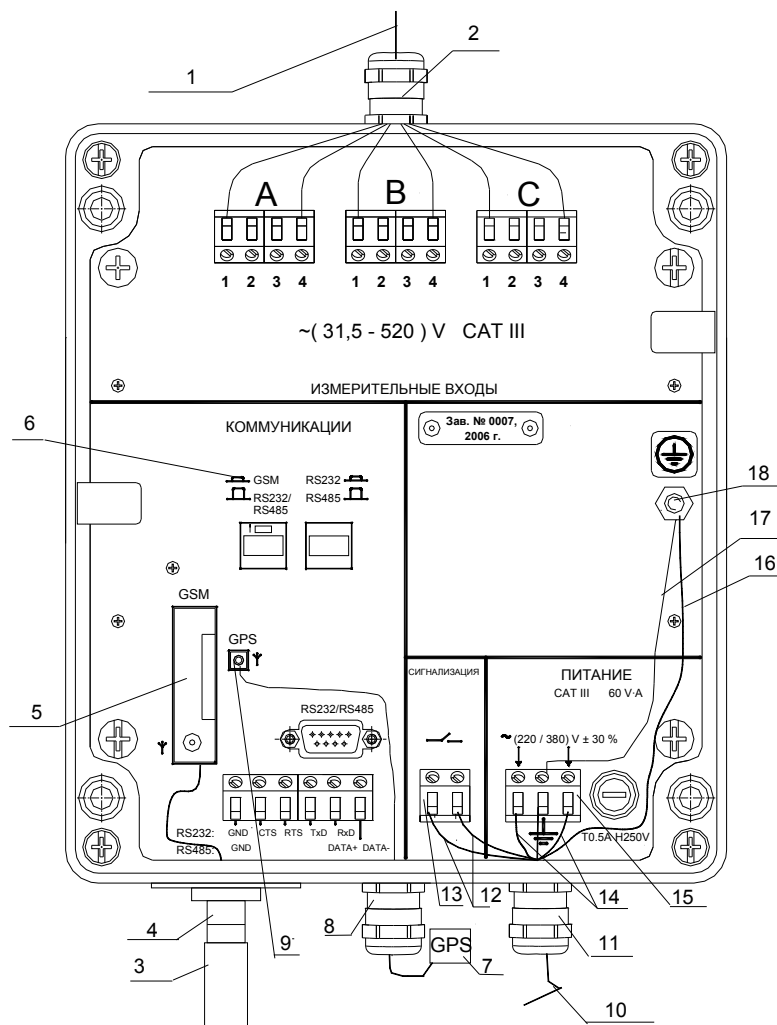
Рисунок А.12 Вариант исполнения и схема подключения регистратора показателей качества электрической энергии «Парма РК3.02» РА1.003.002-011
