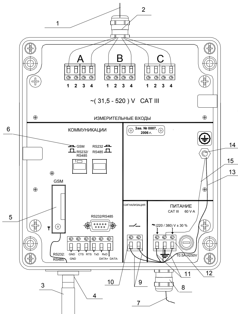
Рисунок А.11 Вариант исполнения и схема подключения регистратора показателей качества электрической энергии «Парма РК3.02» РА1.003.002-010
