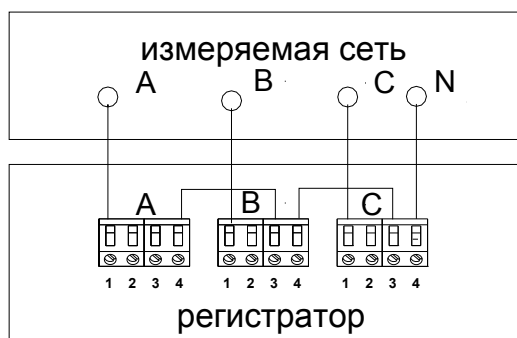
Рисунок 6 Схема подключения измерительных входов регистратора при 4-х проводной схеме подключения
