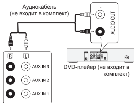
Задняя панель основного устройства
