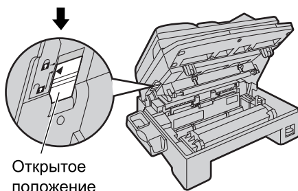
Транспортировочный замок
