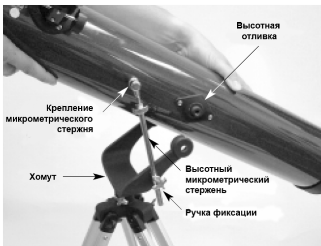
Рисунок 2. Установка оптической трубы в хомут альтазимутального штатива
