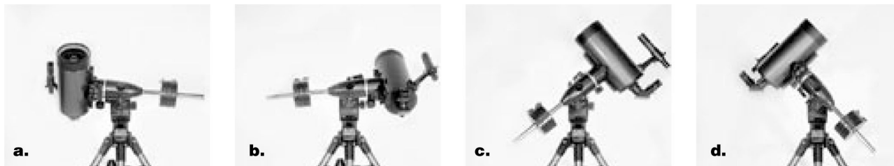
Рисунок 12a-12d. Здесь показан телескоп, ориентированный в четырех направлениях: (a) север, (b) юг, (c) восток, (d) запад. Обратите внимание, что тренога и штатив не должны перемещаться; только труба телескопа должна поворачиваться вокруг осей склонения и прямого восхождения.
