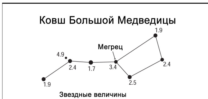
Рисунок 13. Мегрец - звезда, соединяющая ручку ковша с самим ковшем. Это хороший способ определения состояния атмосферы. Если Вы не видите Мегрец, условия для наблюдений плохие.
