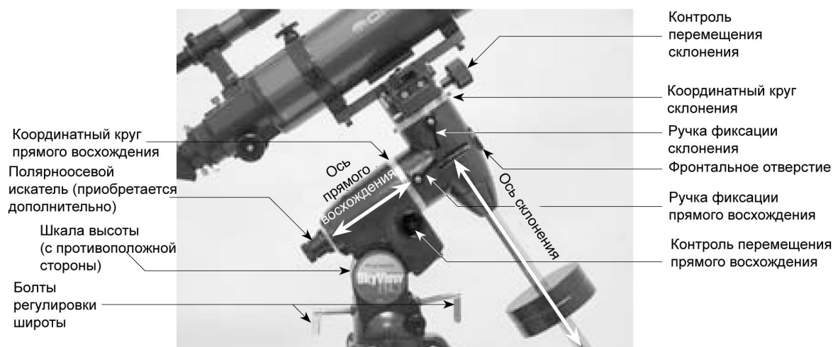
Рисунок 8. Монтировка SkyView Pro.
