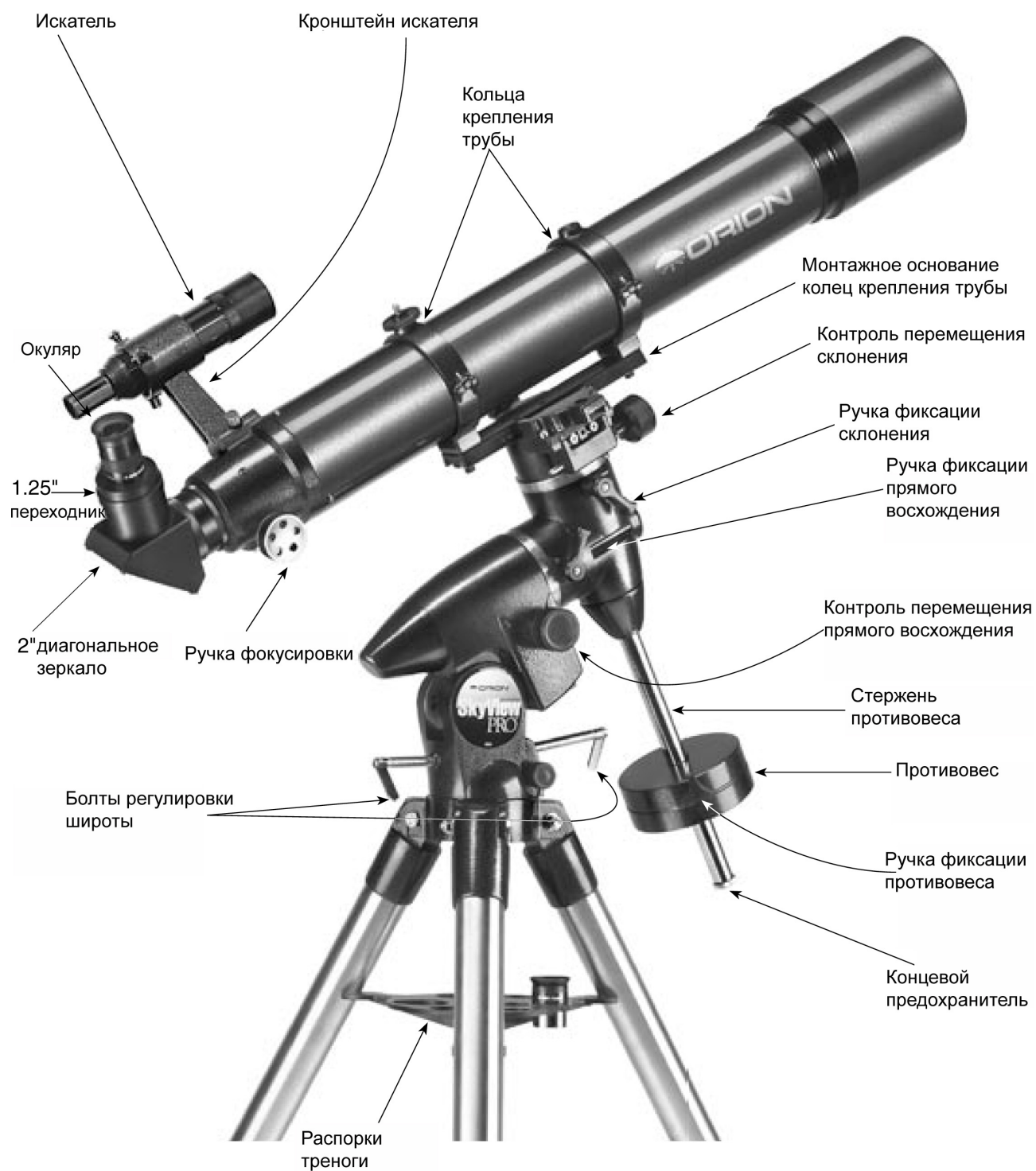
Рисунок 1. Телескоп-рефрактор SkyView Pro 100 мм ED EQ
