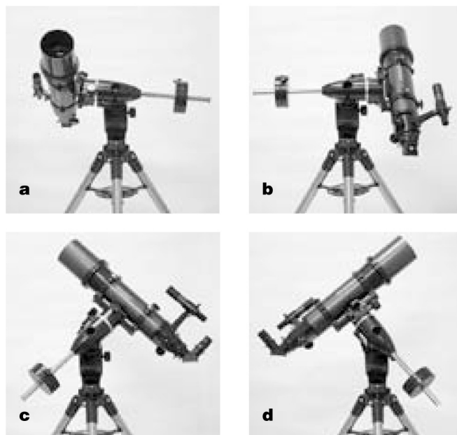
Рисунок 14а-д. Здесь показан телескоп, ориентированный в четырех направлениях (а) север, (b) юг, (с) восток, (d) запад. Обратите внимание, что тренога и монтировка не должны перемещаться; только труба телескопа должна поворачиваться вокруг осей склонения и прямого восхождения.
