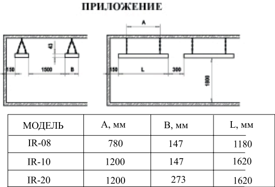
Рис. 1 Схема размещения обогревателя
