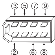
Колодка МК вид спереди, со стороны контактов
