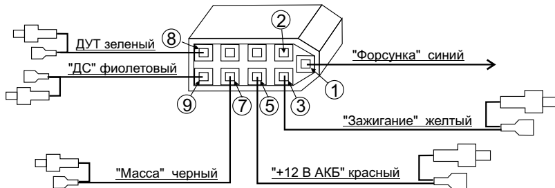
Колодка переходника МК вид сзади со стороны присоединения проводов
