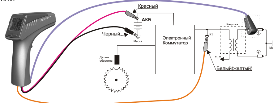
Схема подключения 3
