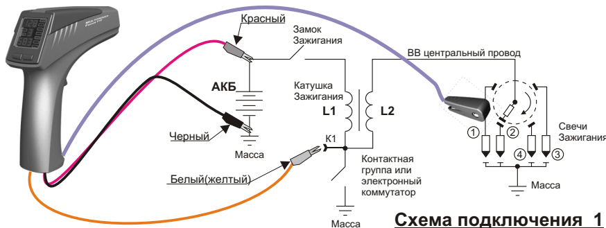
Схема подключения 1
