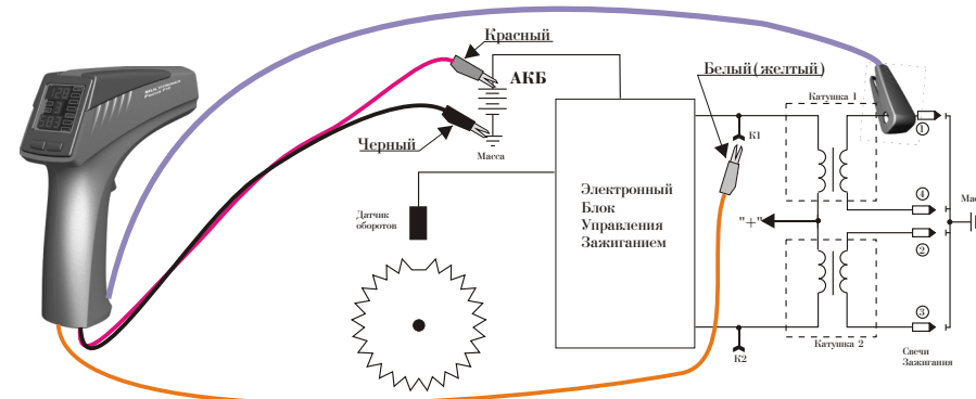
Схема подключения 2
