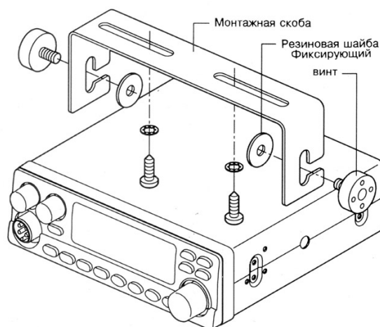
Рис. 1. Крепление радиостанции при помощи монтажной скобы.
