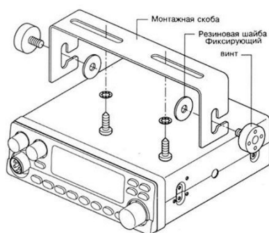
Рис.1. Крепление радиостанции при помощи монтажной скобы.
