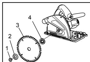
1. Boulon hexagonal 2. Bague externe 3. Lame 4. Flasque intérieur
