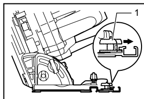
1. Levier coulissant
