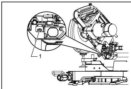
1. Skrūve, kas nostiprina lāzera iekārtas korpusu 014275
