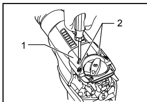
1. Cubierta de la tapa del cárter 2. Tornillos
