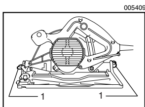
1. Зажимной винт
