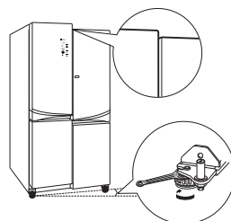
3 Выравнивание положения холодильника и двери
