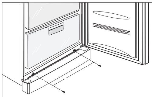
Рис 1. Установка нижней декоративной панели. (Для моделей GA**409Q***)
