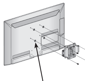
4-Кольцевые уплотнители
