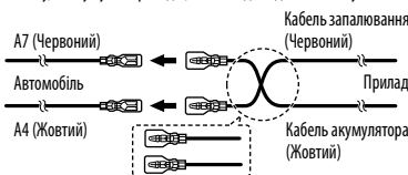
Стандартний варіант схеми підключення проводів
