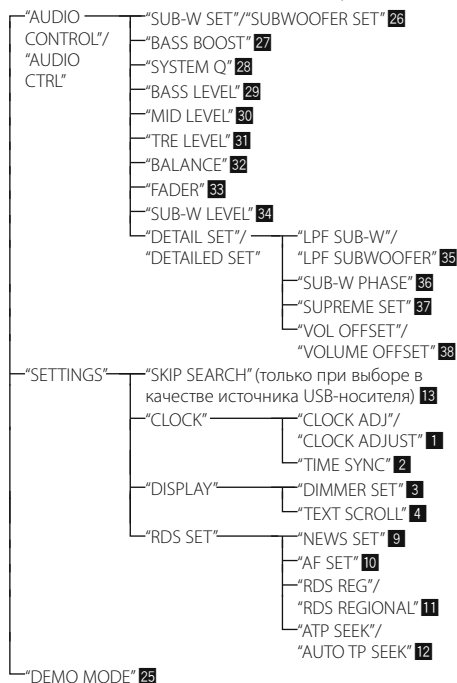
Функциональные элементы, отображаемые при выборе в качестве источника проигрывателя компакт-дисков и аудиофайлов
