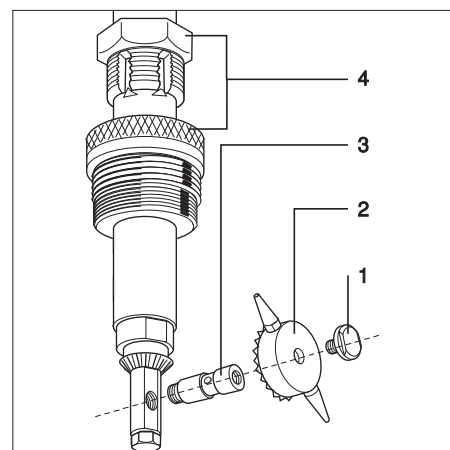
1 Резьбовая пробка
