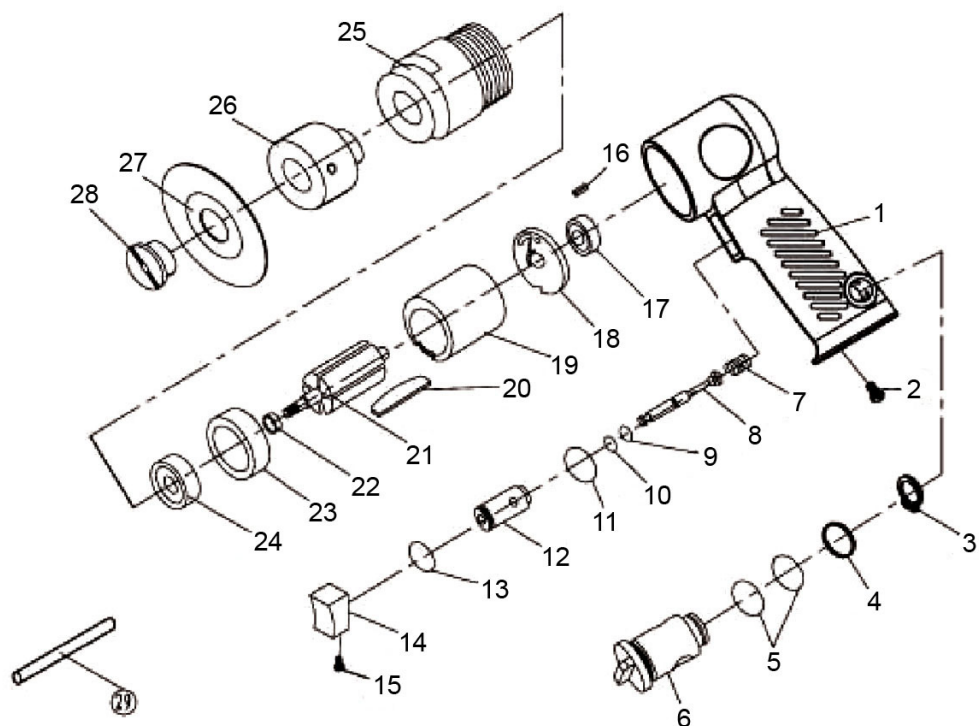
Рис. 3. Схема шлифмашины модели ПМШУ - 6,3/ 125 ПТ
