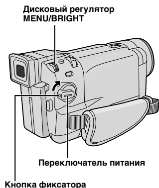
Кнопка фиксатора
