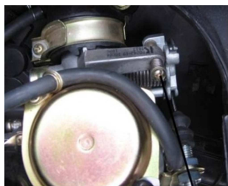
Регулировочный винт
