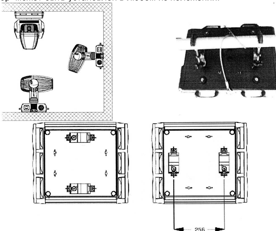
Установка монтажных скоб.
