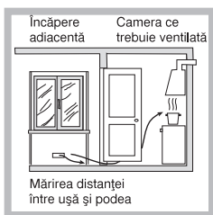
Exemple de deschidere (fante) pentru aerisire
