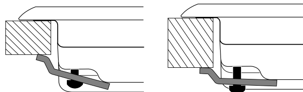
Poziția clemei pentru sus H=20mm
