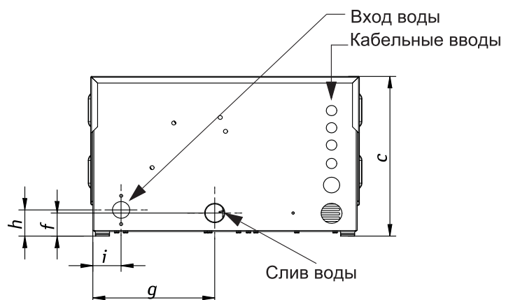
Вид снизу
