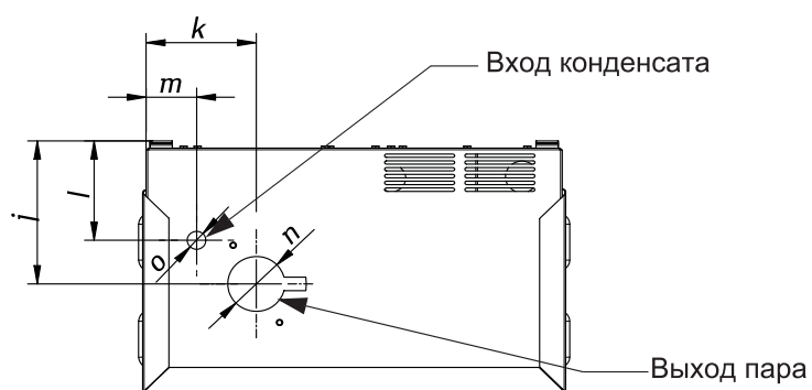
Вид сверху
