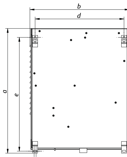
Вид сзади
