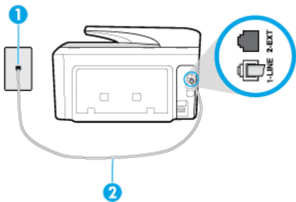
Рисунок 5-5 Вид принтера сзади
