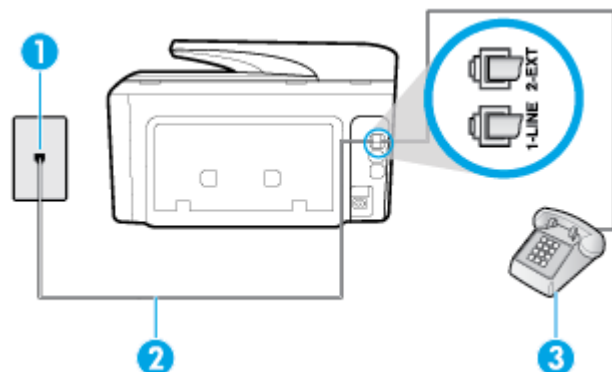
Рисунок 5-4 Вид принтера сзади
