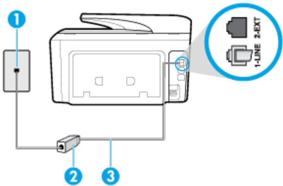
Рисунок 5-2 Вид принтера сзади
