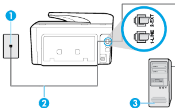
Рисунок 5-6 Вид принтера сзади
