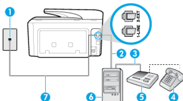
Рисунок 5-13 Вид принтера сзади
