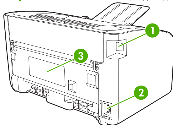
Рисунок 1-2 HP LaserJet P1000, вид сзади (изображена модель HP LaserJet P1006/P1009)
