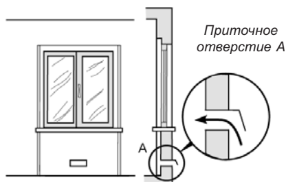
Пример обеспечения притока воздуха
