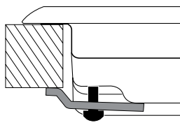
Монтаж крюка для опорных брусков H=30mm
