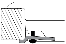
Монтаж крюка для опорных брусков H=40mm
