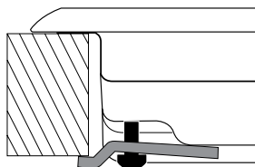
Ілмек орны шкаф үстінің қалыңдығы H=40\text{мм} үшін
