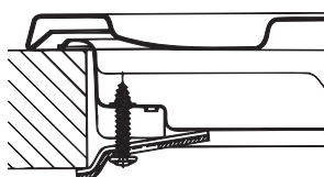
Poziția clemei pentru sus H=40mm
