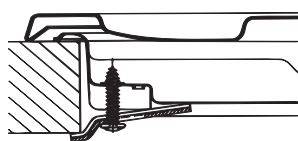
Монтаж крюка для опорных брусков H=40mm
