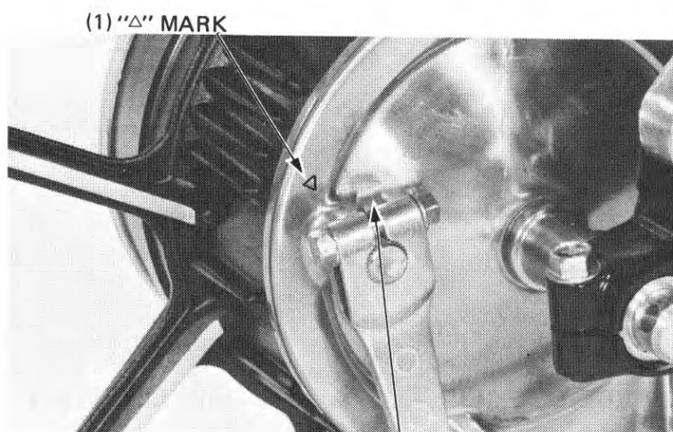
(2) ARROW
