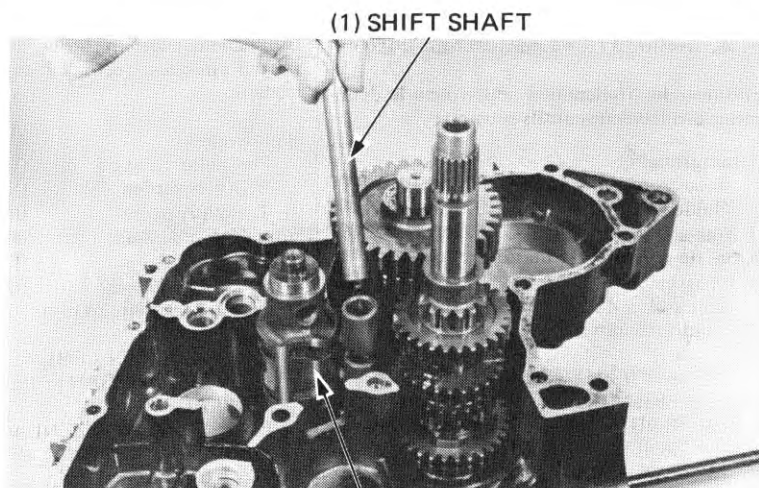
(2) SHIFT DRUM
