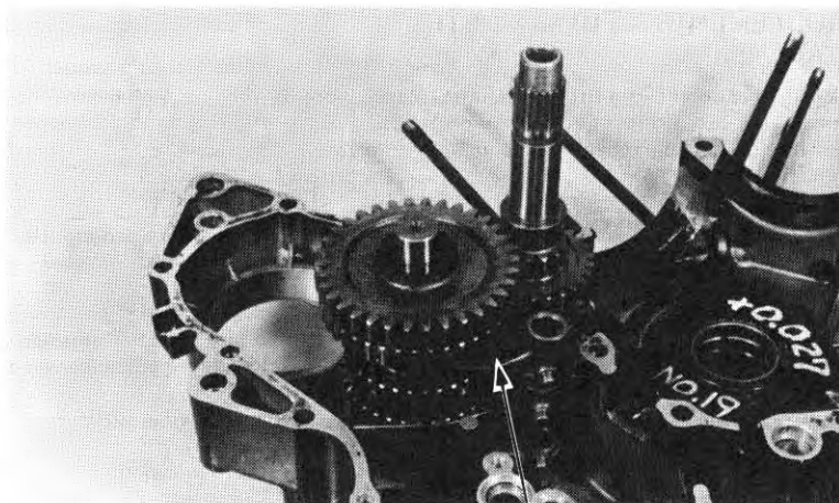
(1) MARK
