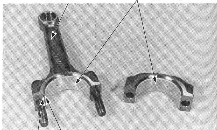
(3) GROOVE (4) BOSS
