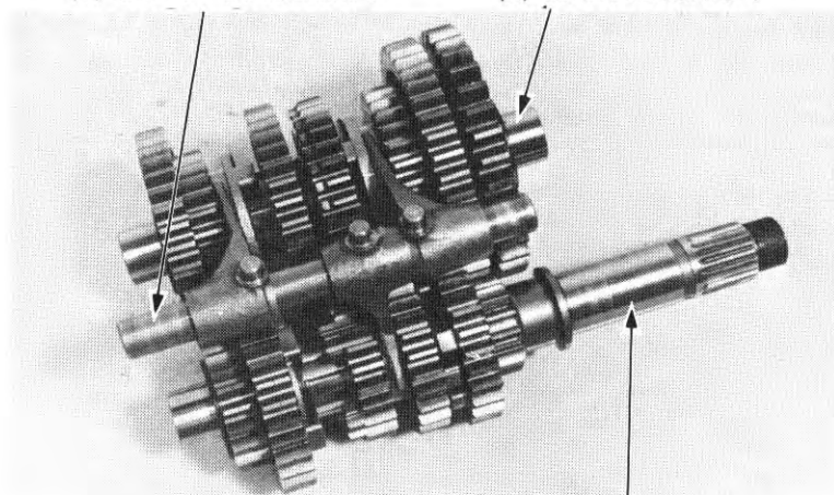
(3) MAINSHAFT
