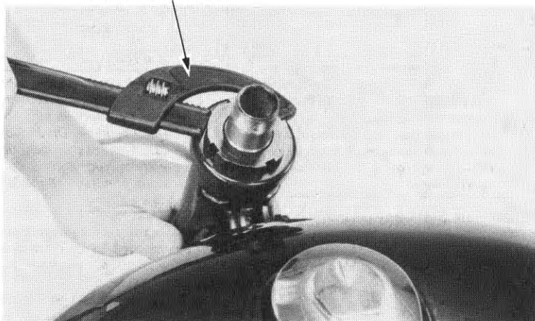
(1) PIN SPANNER
