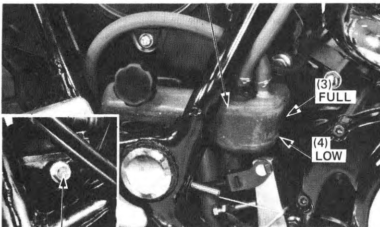
(2) BLEED BOLT
