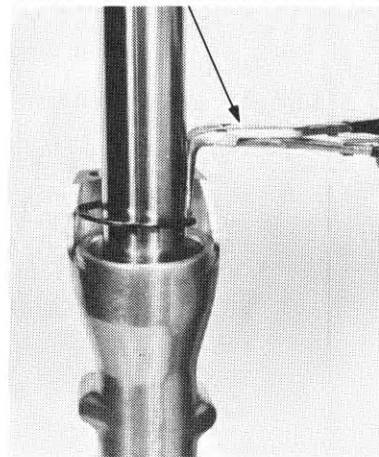
(1) SNAP RING PLIERS 07914-3230001
