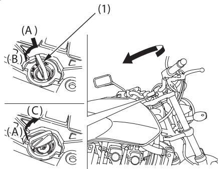
(1) Ключ зажигания
