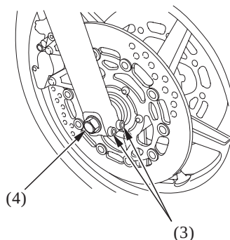
(4) Осевой болт
