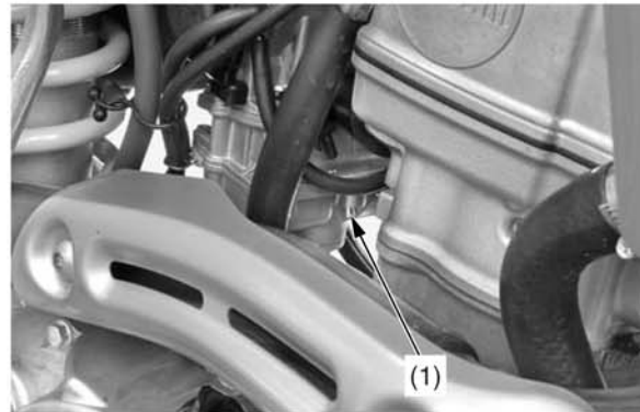
(1) винт регулировки частоты вращения вала двигателя на холостом ходу
