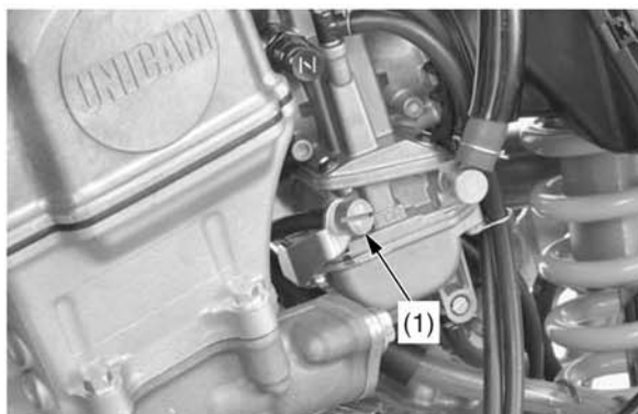
(1) винт ограничения угла закрытия дроссельной заслонки
