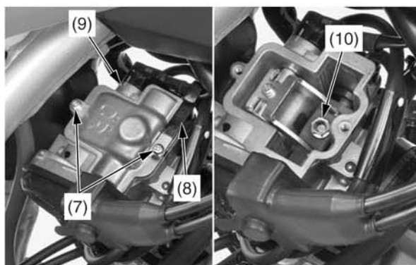
(7) винты верхней части карбюратора (8) хомут троса (9) верхняя часть карбюратора (10) игла распылителя/держатель в сборе
