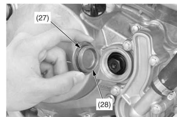
(27) уплотнительное кольцо (28) пробка контрольного отверстия коленчатого вала
