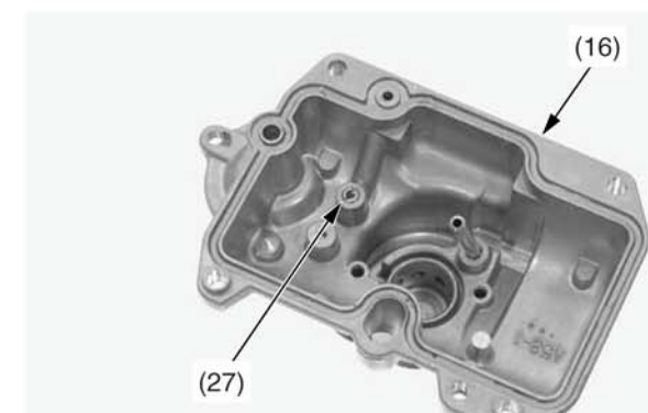
(16) поплавковая камера (27) обратный жиклер
