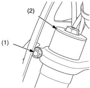
(1) верхние стяжные болты (2) наконечник вилки
