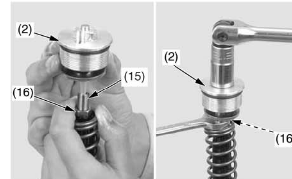
(2) наконечник вилки (15) поршневой шток (16) контргайка
