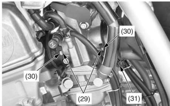
(29) фиксаторы (30) канавки (31) винт хомута соединительной трубки
