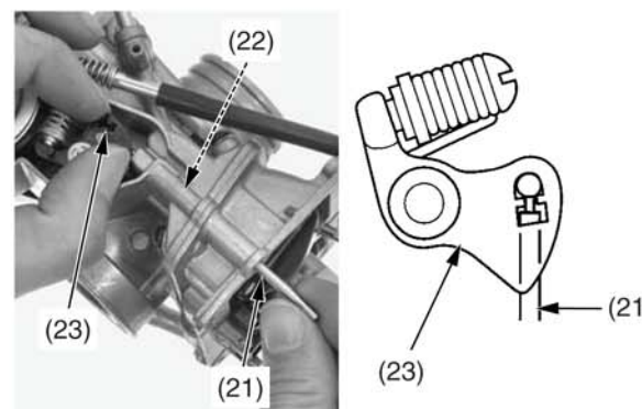
(21) шток плунжера (22) канал штока (23) рычаг
