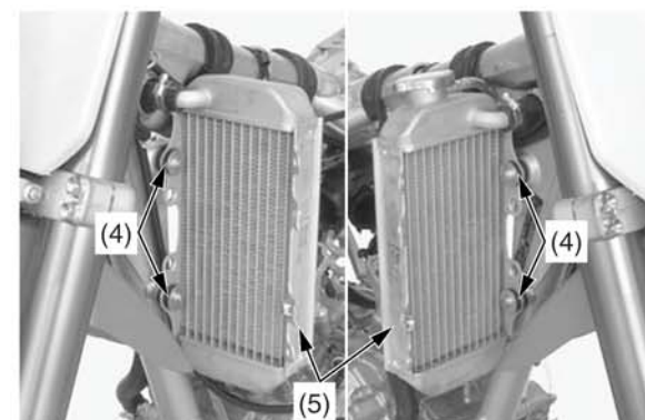
(4) крепежные болты радиаторов и их шайбы (5) радиаторы
