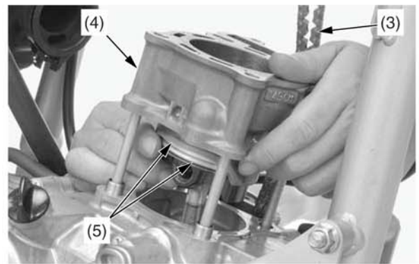
(3) цепь распредвала (4) цилиндр (5) поршневые кольца
