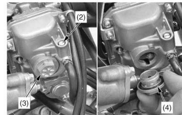
(2) винт сливного отверстия
