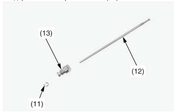
(11) фиксатор (12) игла клапана (13) держатель иглы распылителя
