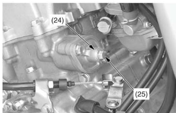
(24) уплотнительная шайба (25) болт кожуха натяжного ролика цепи распределительного вала
