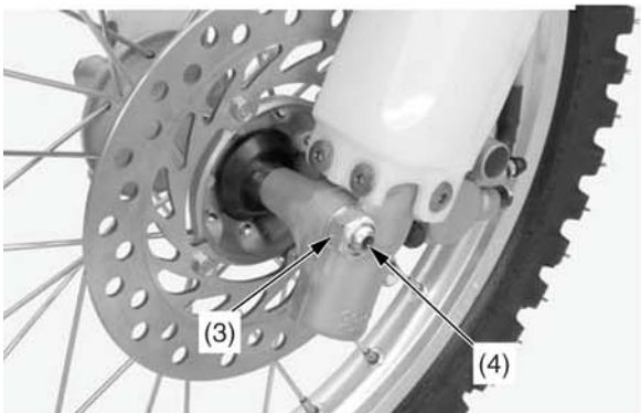
(3) гайка оси (4) ось переднего колеса
