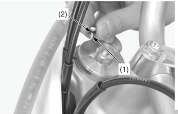
(1) винт стравливания давления (2) уплотнительное кольцо
