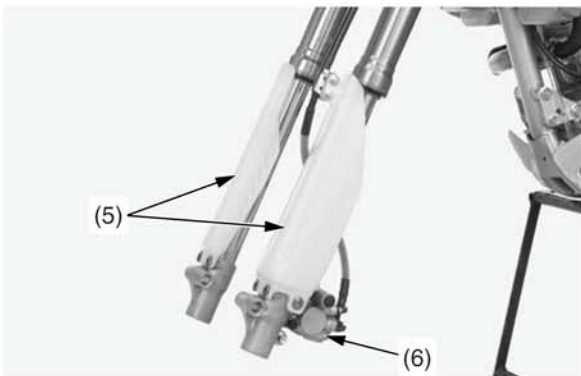
(5) грязевые щитки вилки (6) тормозной суппорт
