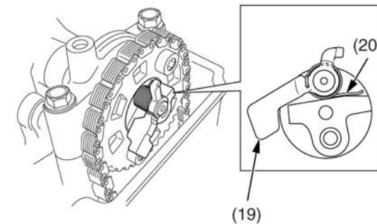
(19) грузик декомпрессора (20) возвратная пружина
