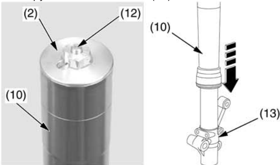
(2) наконечник вилки (10) труба вилки (12) регулировочный винт (13) нижний торец внешней трубчатого наконечника
