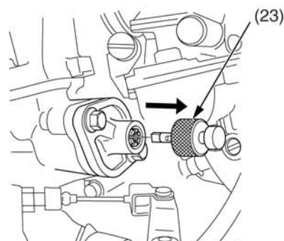
(23) стопор натяжителя
