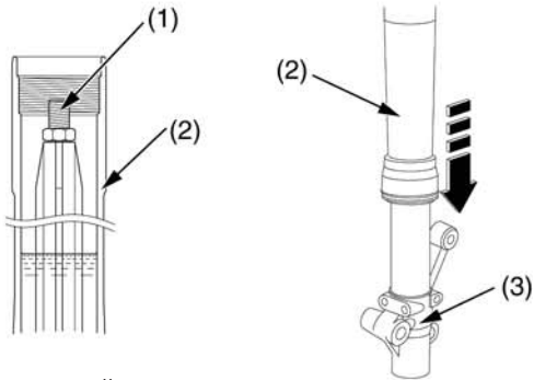
(1) поршневой шток (2) труба вилки (3) нижняя часть внешней трубы вилки
