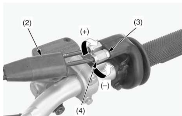
(2) противопылевой колпачок
