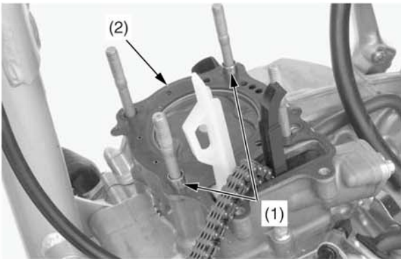
(1) установочные шпильки (2) прокладка головки цилиндра
