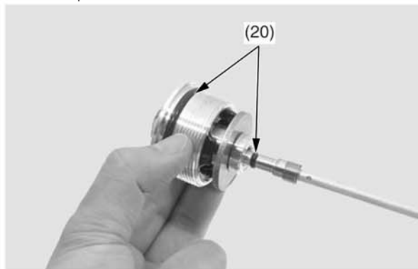
(20) уплотнительные кольца
