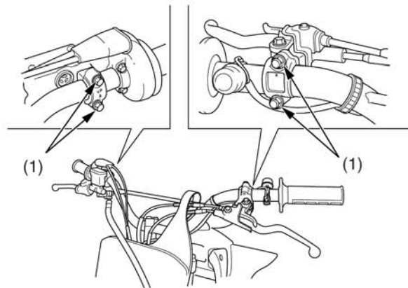
(1) крепежные болты рычагов управления
