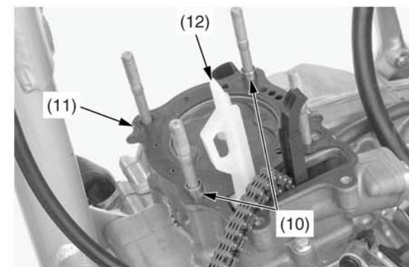
(10) установочные шпильки (11) прокладка головки цилиндра (12) направляющая цепи распредвала
