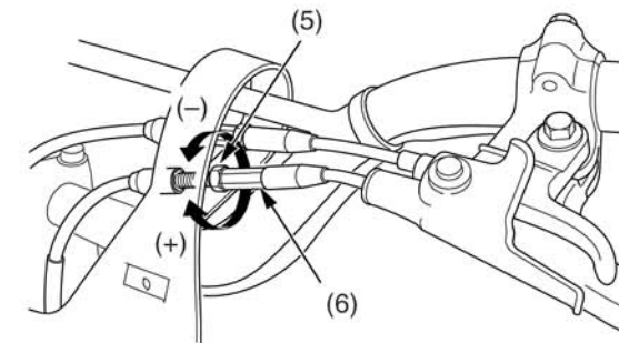
(5) контргайка (6) интегральный регулятор троса акселератора (+) увеличить (-) уменьшить
