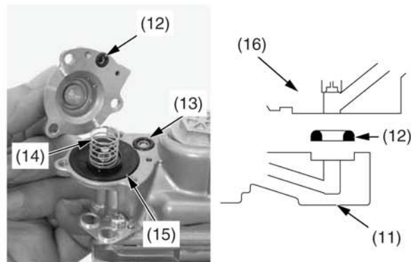
(11) крышка ускорительного насоса (12) U-образное уплотнительное кольцо (13) уплотнительное кольцо круглого сечения (14) пружина (15) диафрагма (16) поплавковая камера
