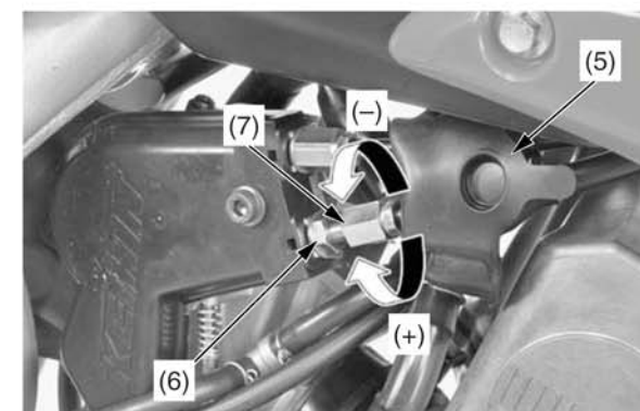
(5) противопылевой колпачок
