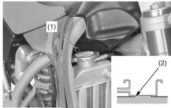
(1) крышка горловины радиатора (2) заправочная горловина
