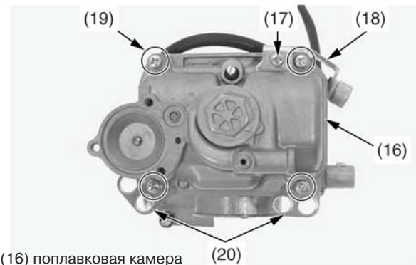
(16) поплавковая камера (17) винт держателя (18) винт держателя ограничителя угла закрытия дроссельной заслонки (19) винты поплавковой камеры (20) направляющие шлангов
