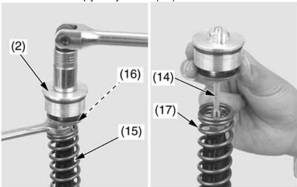
(2) наконечник вилки (14) игольчатый шток регулятора (15) поршневой шток (16) контргайка (17) пружина вилки
