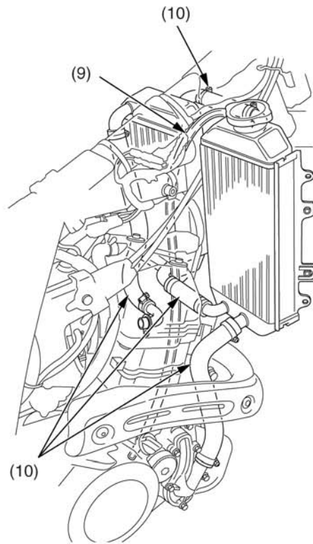
(9) дренажная трубка радиатора (10) магистрали системы охлаждения
