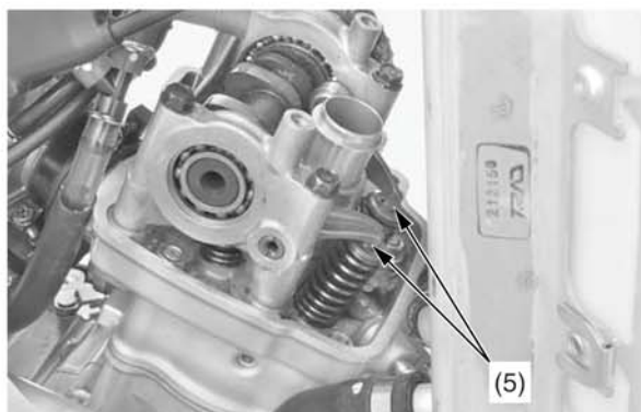
(5) коромысла выпускных клапанов
