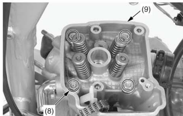
(8) гайки головки цилиндра и их шайбы (9) головка цилиндра
