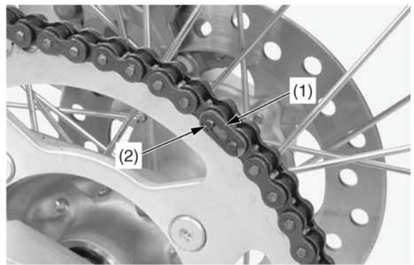
(1) чека (2) соединительное звено
