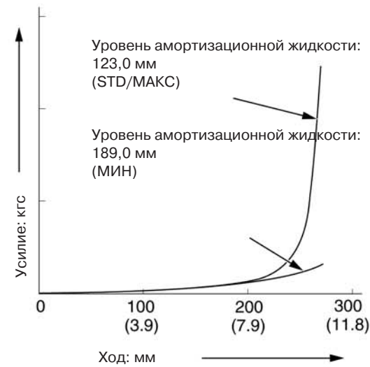
Характеристики хода подвески
