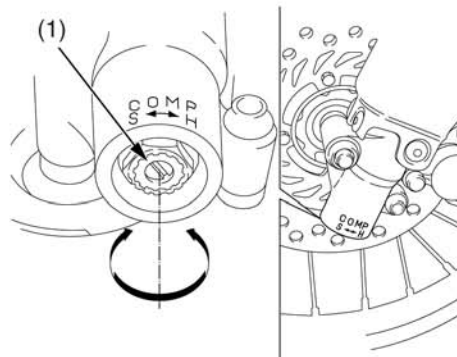
(1) регулятор демпфирующего усилия сжатия
