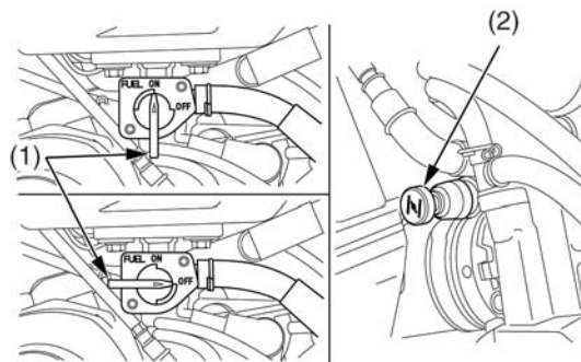
(1) топливный кран (2) рукоятка воздушной заслонки
