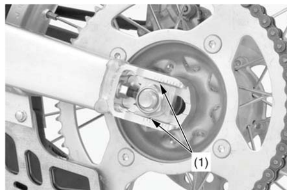
(1) регулировочная метка
