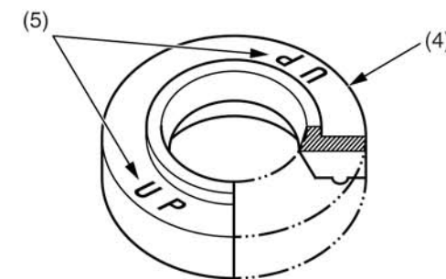
(4) резиновая прокладка (5) метки "UP"
