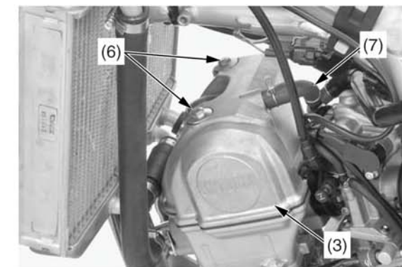
(3) крышка головки цилиндра (6) болты крышки головки цилиндра (7) вентиляционная трубка
