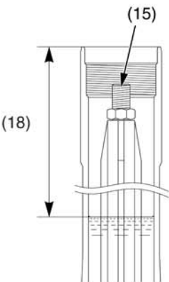
(15) поршневой шток (18) уровень масла
