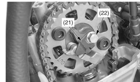
(21) стопорная пластина 22 болт (продолжение на следующей странице)
