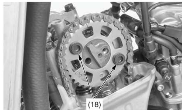
(18) болты звездочки распределительного вала
