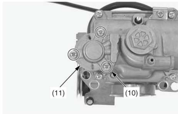
(10) винты крышки ускорительного насоса (11) крышка ускорительного насоса
