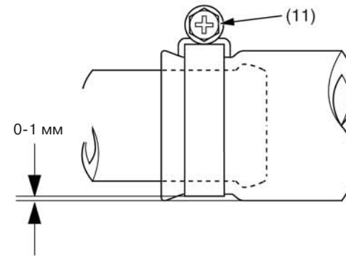
(11) винт хомута трубопровода
