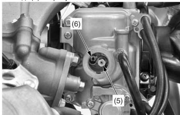
(5) главный жиклер (6) жиклер холостого хода
