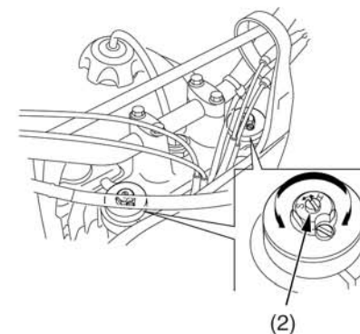
(2) регулятор демпфирующего усилия отбоя
