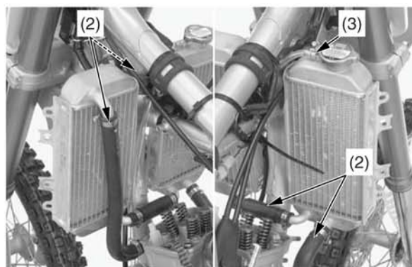
(2) магистрали системы охлаждения (3) дренажная трубка радиатора
