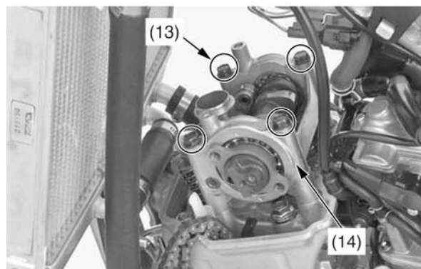
(13) болты узла держателя распределительного вала (14) держатель распределительного вала в сборе
