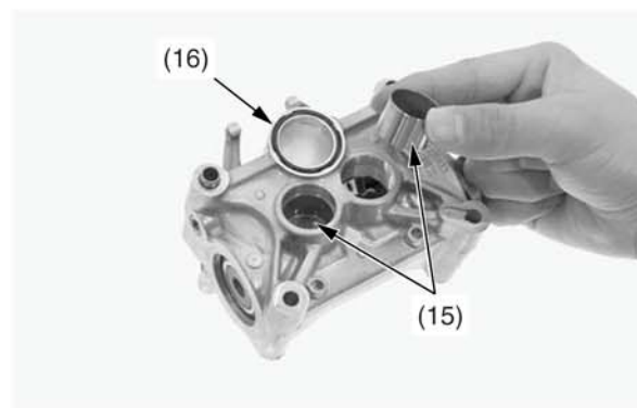
(15) толкатели клапанов (16) уплотнительное кольцо
