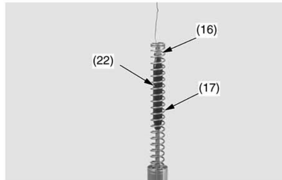
(16) контргайка (17) пружина вилки (22) направляющая пружины
