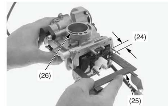
(24) верхнее положение поплавка (25) поплавковый уровнемер (26) впускное окно
