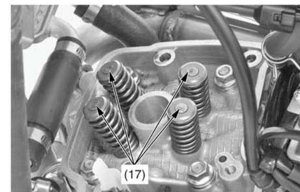
(17) регулировочные шайбы
