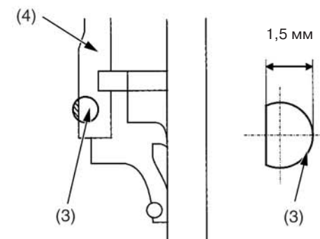
(3) изнашиваемая втулка (4) внешняя труба
