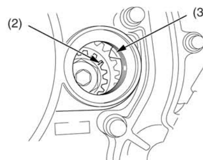
(2) установочная линия (3) установочная метка
