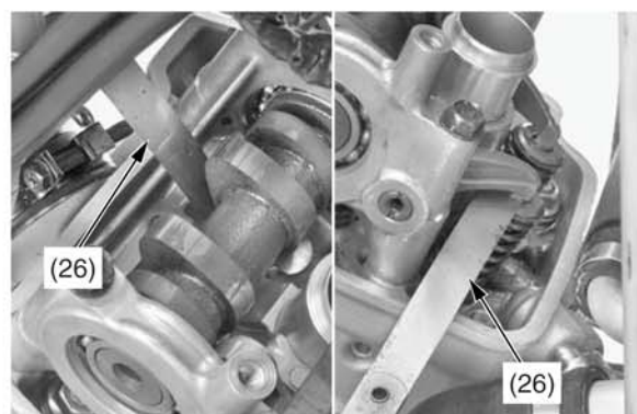
(26) калибр для измерения зазоров
