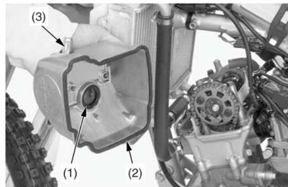
(1) уплотнение гнезда свечи зажигания (2) прокладка крышки головки цилиндра (3) крышка головки цилиндра
