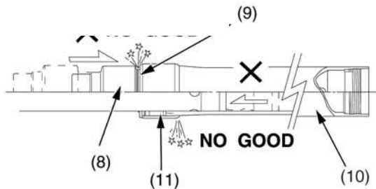
(8) трубчатый наконечник (9) сальник (10) труба вилки (11) направляющая втулка
