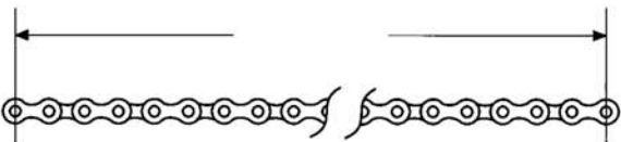
ИЗМЕРЬТЕ ДЛИНУ 21 ЗВЕНА ПРИВОДНОЙ ЦЕПИ
