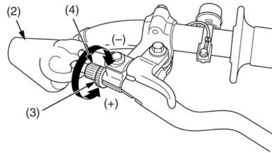
(2) противопылевой колпачок (3) контргайка (4) регулятор троса (+) увеличить (-) уменьшить
