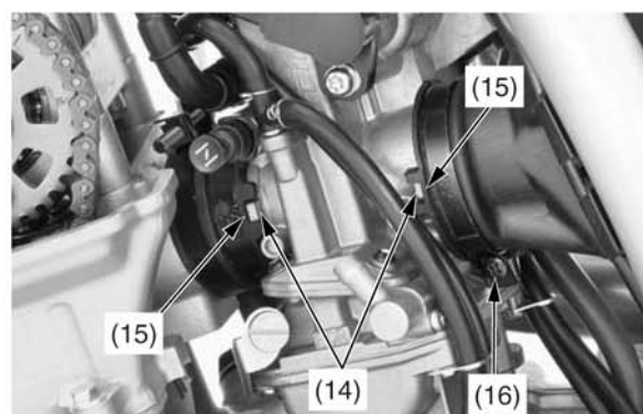
(14) фиксаторы (15) канавки (16) винт хомута соединительной трубки
