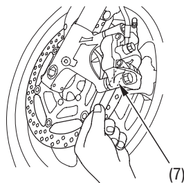
(6) Зазор (7) Щуп-калибр
