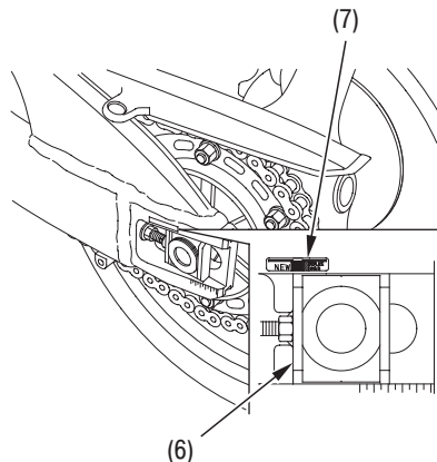
(6) Регулировочная пластина
