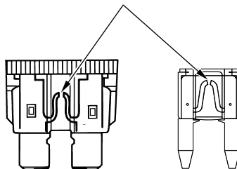
Перегоревший предохранитель
