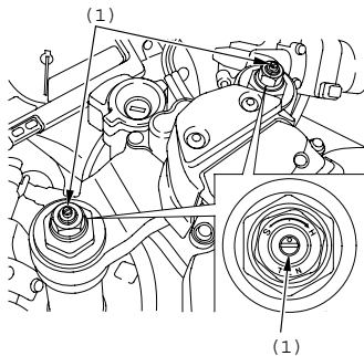
(1) Регулятор демпфирующего усилия
