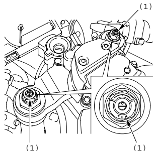
(1) Регулятор предварительного сжатия пружины
