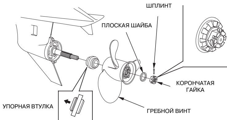
Гребной винт
