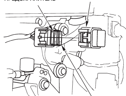
ПРЕДОХРАНИТЕЛЬ 15 А
