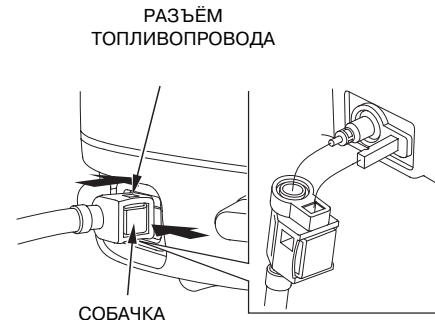
(СО СТОРОНЫ ПОДВЕСНОГО МОТОРА)
