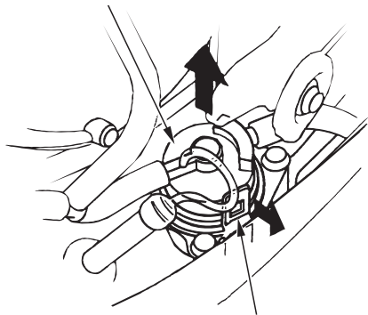
ПРУЖИННЫЙ ФИКСАТОР
