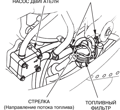
ХОМУТЫ
